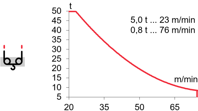
EC3075VF 22 kW
