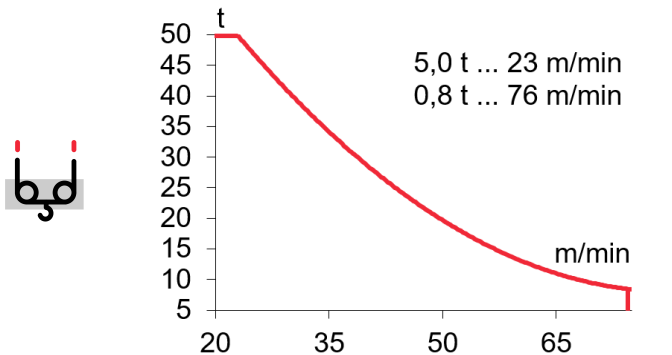
EC3075VF 22 kW
