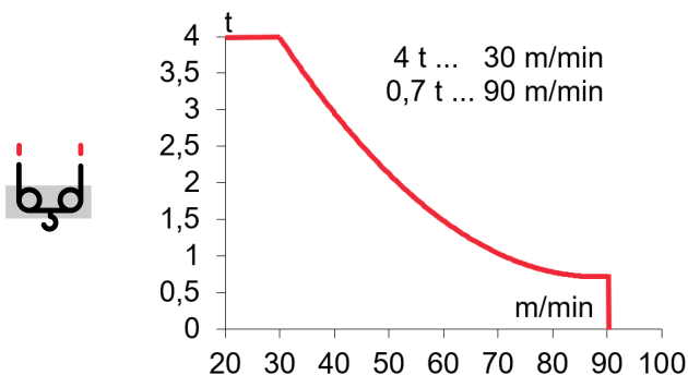
EC3090VF 22 kW
