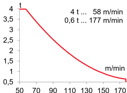
*EC60180VF 45 kW
