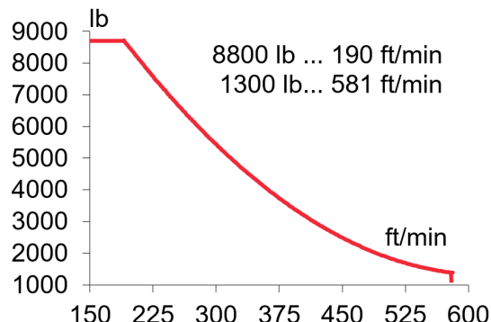
*EC60180VF 45 kW
