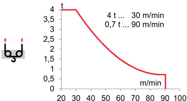
EC3090VF 22 kW
