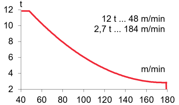
* EC150185VF 110 kW
