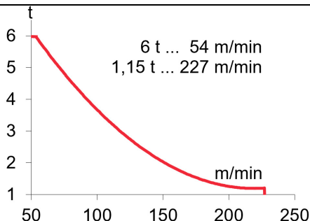
* EC88227VF 65 kW
