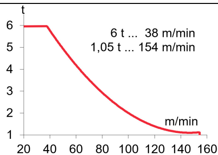
EC60154VF 45 kW
