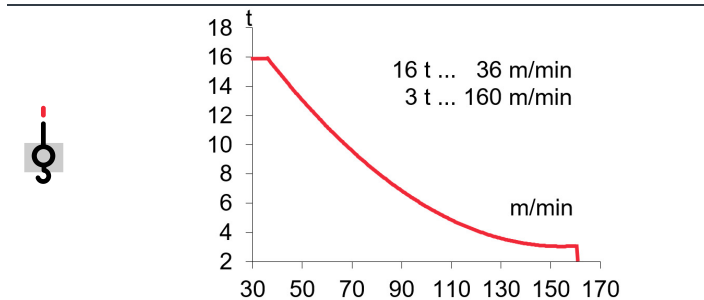
EC150160VF 110 kW
