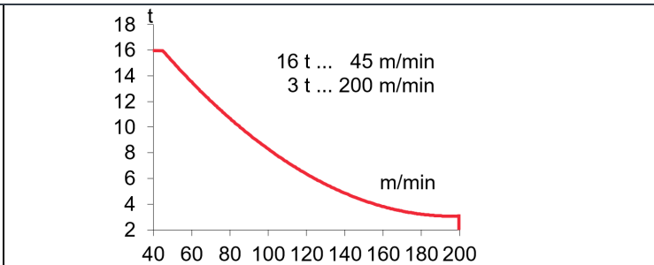
* EC180200VF 132 kW
