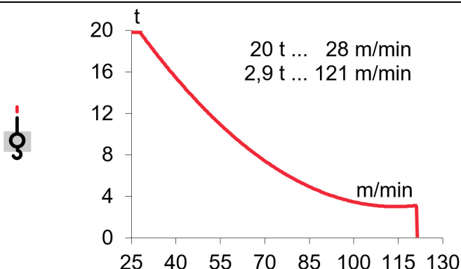
EC150120VF 110 kW
