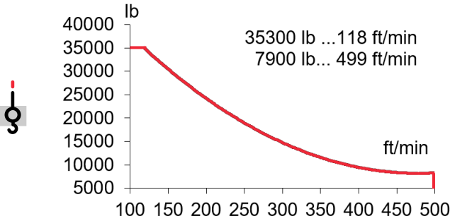
EC150152VF 110 kW
