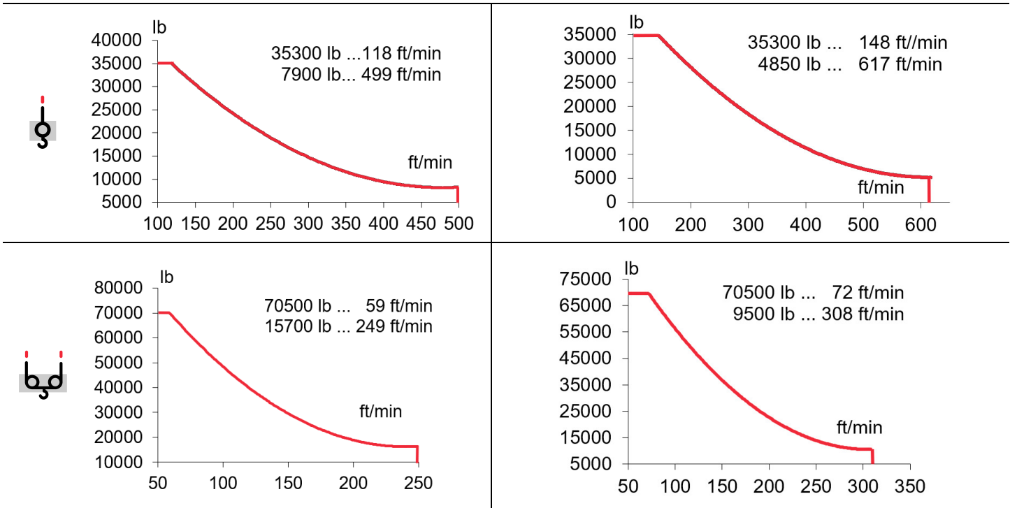
EC150152VF 110 kW
