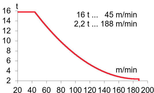
* EC180188VF 132 kW
