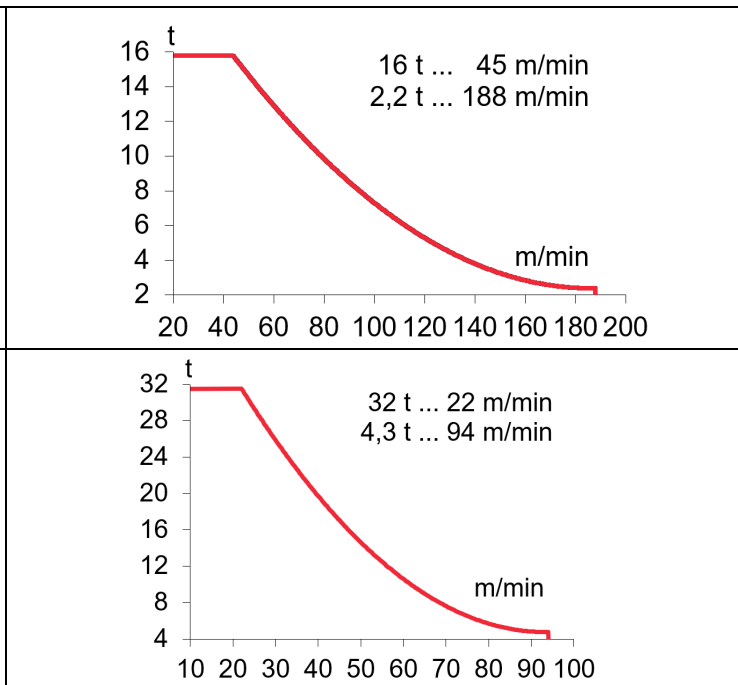
* EC180188VF 132 kW
