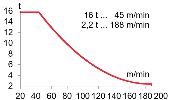
* EC180188VF 132 kW
