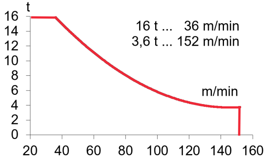
EC150152VF 110 kW
