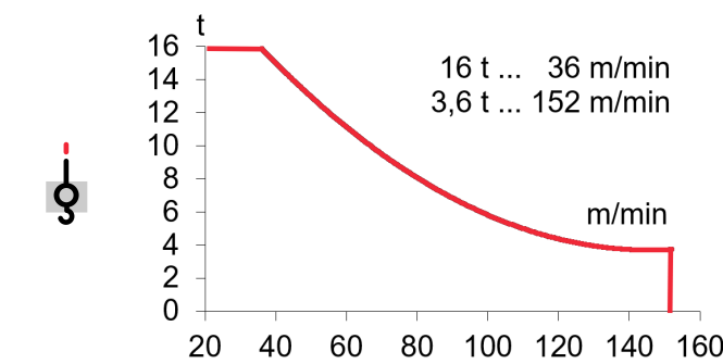
EC150152VF 110 kW
