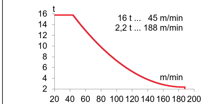
* EC180188VF 132 kW
