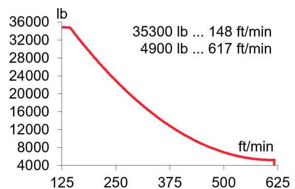
* EC180188VF 132 kW
