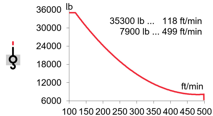
EC150152VF 110 kW
