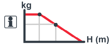
TG4025VF 4 x 7,5 kW
